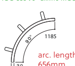
RINGO 835 90° 3xM10 MODULE
